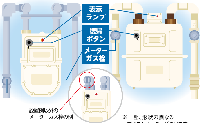
家庭用マイコンメーター設置例
