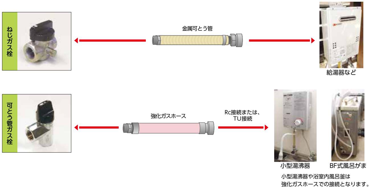
旧型ガス栓
