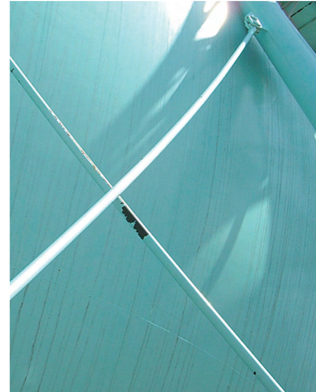
▲球形ガスホルダーは支柱アンカーボルトの伸び（最大 10mm 程度）のほか、支柱タイロッドブレードの伸びやズレが多数発生した。
